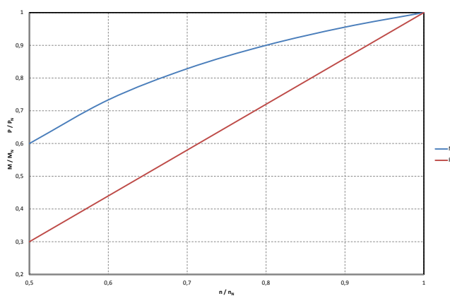
Рис. 2 Снижение мощности и момента с помощью USK
