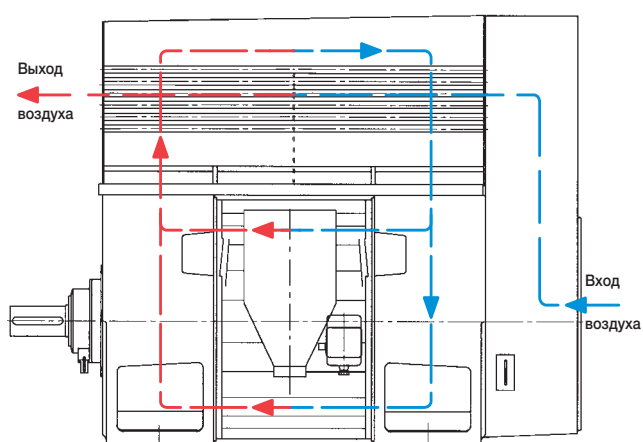
аксиально вентилируемый двигатель с охлаждением «воздух-воздух»
