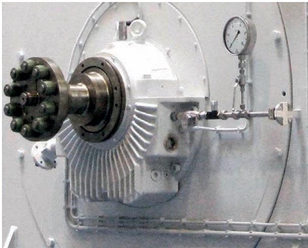
Приспособление для замыкания коротко обмотки ротора и подъема щеток
