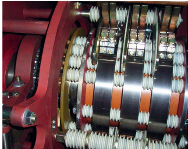
Приспособление для замыкания коротко обмотки ротора и подъема щеток
