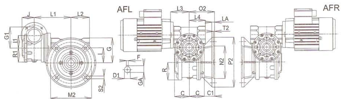
Таб. 12.9 Чертежи размеров
