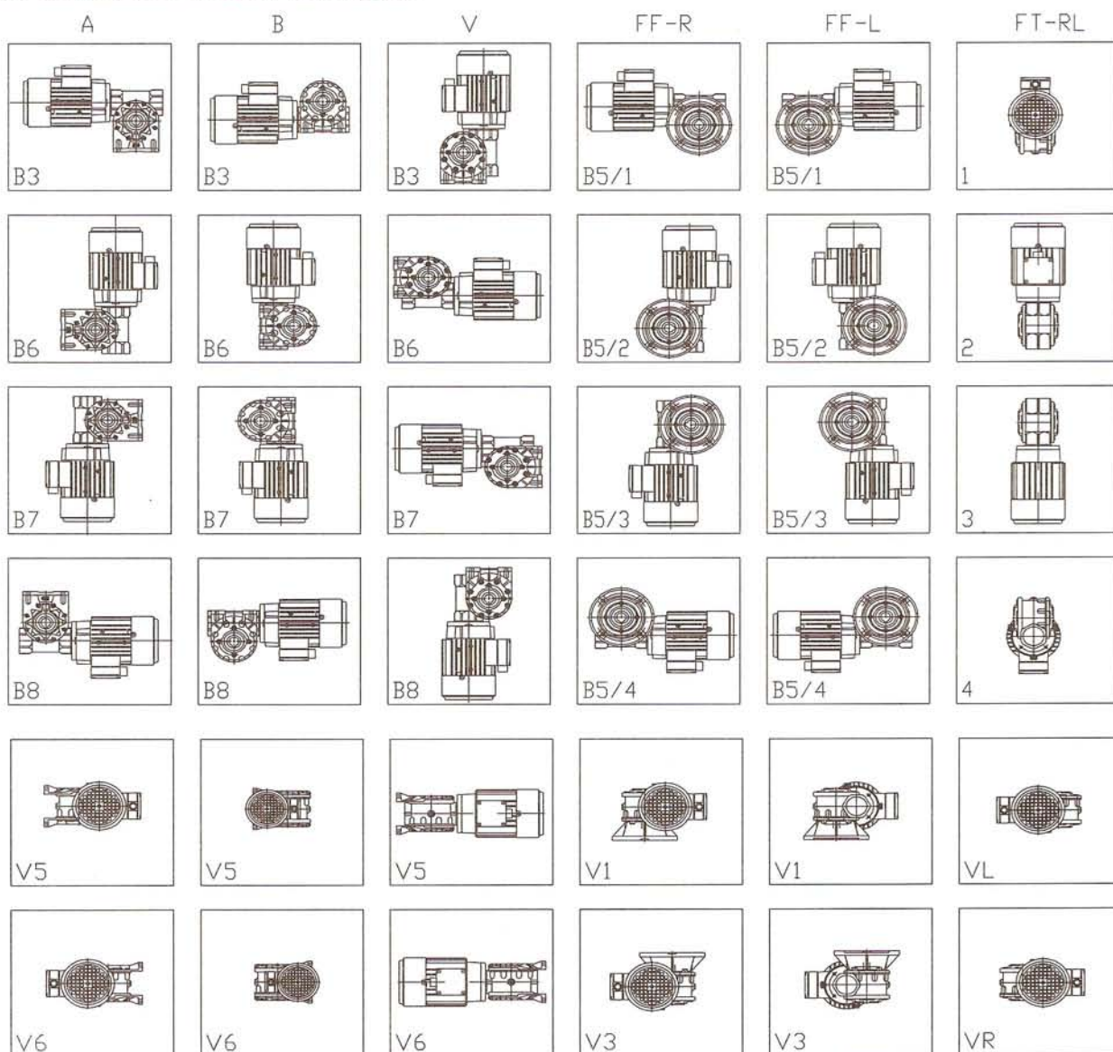
Таб. 3.1 Монтажные позиции и исполнения:
