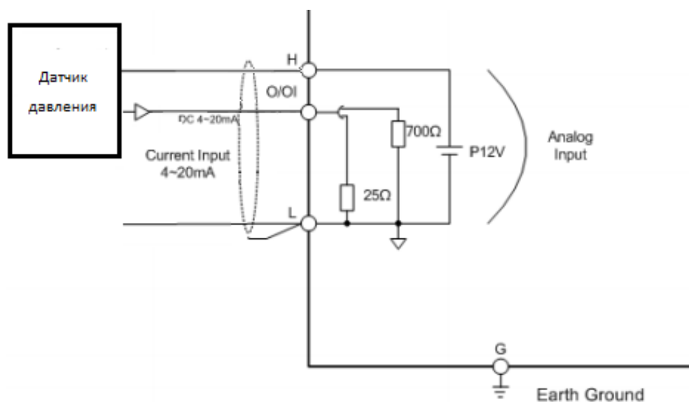
Подключение датчика обратной связи 4..20mA.
