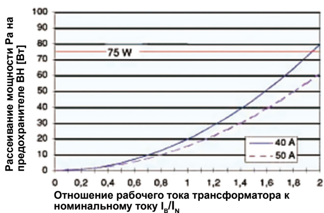
Рис. 9 Рассеивание мощности высоковольтных предохранителей 40 А и 50 А для трансформатора 20 кВ, 630 кВА
