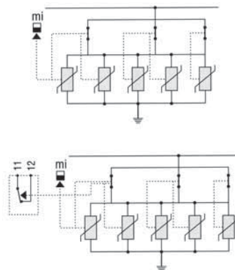
схема соединений
