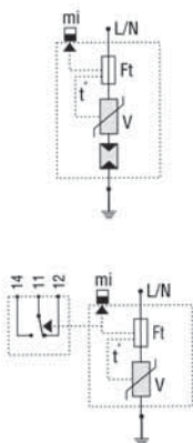
схема соединений
