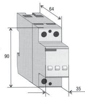
габаритный чертёж
