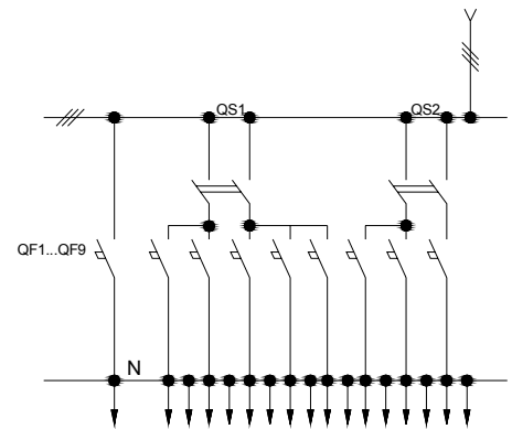
Рис.5.24 (Схема БОУ-46).
