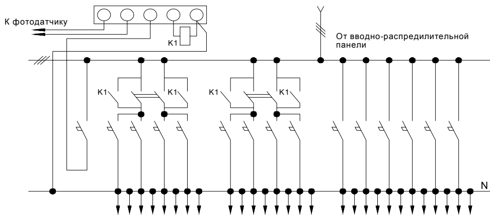
Рис.5.21 (Схема БОУ-43).
