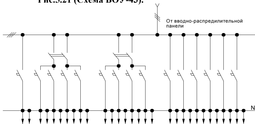
Рис.5.22 (Схема БОУ-44).
